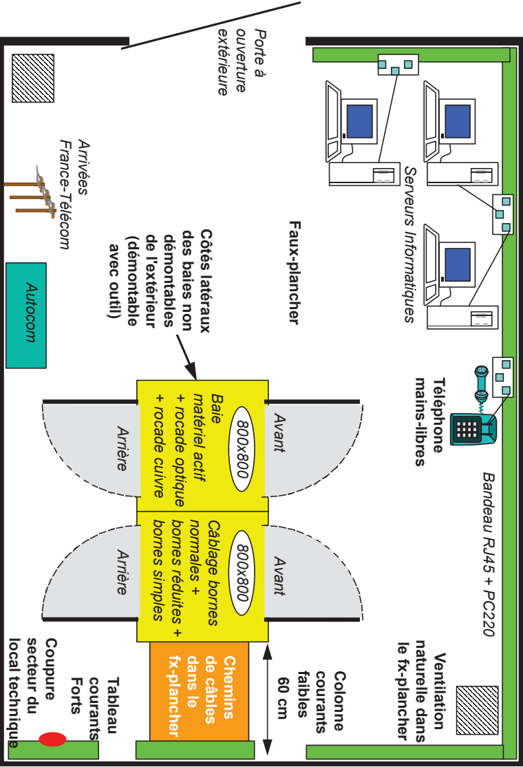
Figure 3 : Exemple d'organisation du local technique principal
